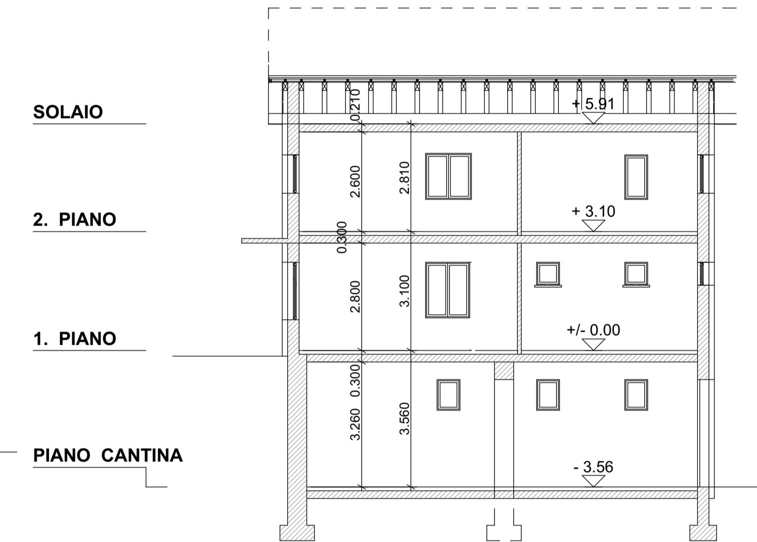
SEZIONE B-B
