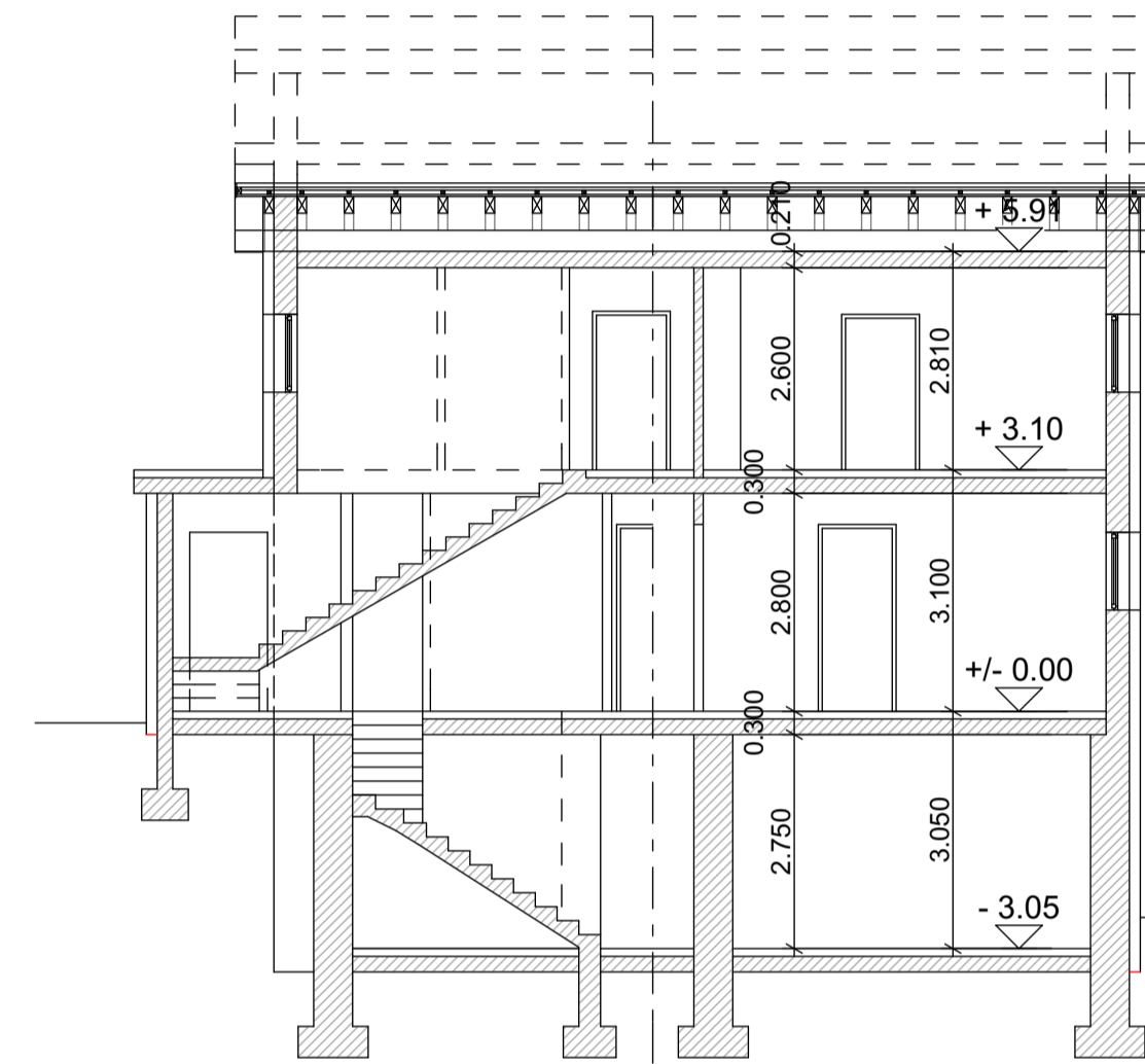
SEZIONE A-A
